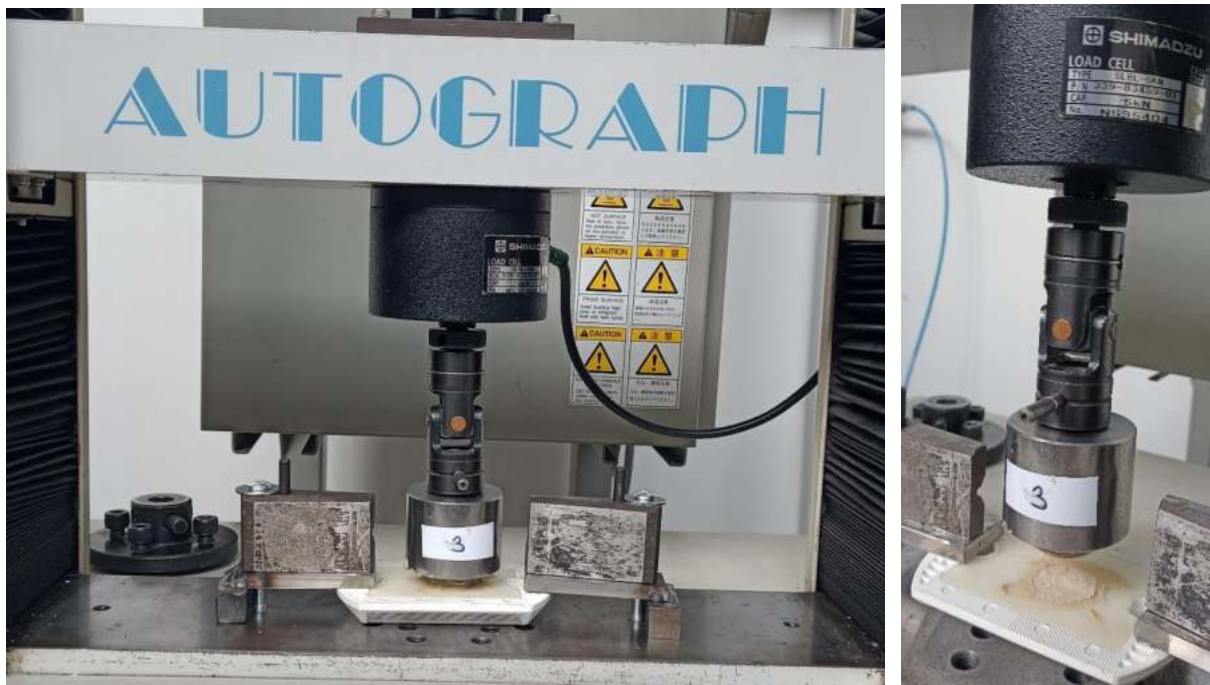
Figura 1. Instalación de una de las muestras para el ensayo
