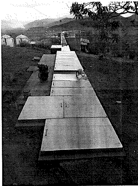
FOTOGRAFIA 3 Y 4: TAPAS EN ACERO INOXIDABLE CALIBRE 18 Y ESTRUCTURA PERIMETRA EN ANGULO DE 11/2"X1/8" REFERENCIA 304.
