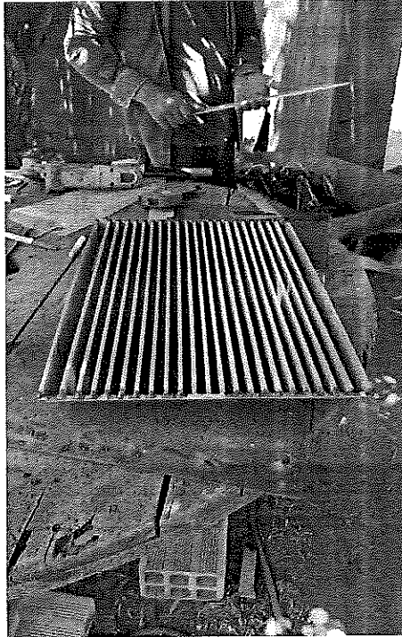
FOTOGRAFIA 1 Y 2: PROCESO DE CONSTRUCCION E INTALACION REJAS DE CRIBADO
