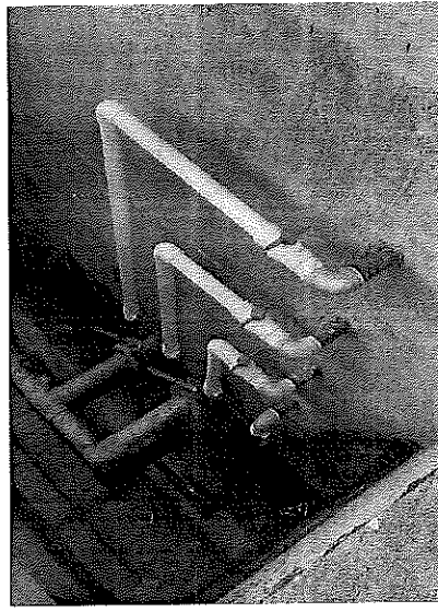
FOTOGRAFIA 9 Y 10: TOMAS DE MUESTRAS DE LODOS CONSTRUIDAS PARA LOS 4 TANQUES.
