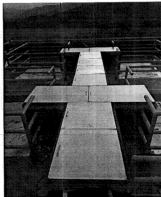
FOTOGRAFIA 3 Y 4: TAPAS EN ACERO INOXIDABLE CALIBRE 18 Y ESTRUCTURA PERIMETRA EN ANGULO DE 11/2"X1/8" REFERENCIA 304.
