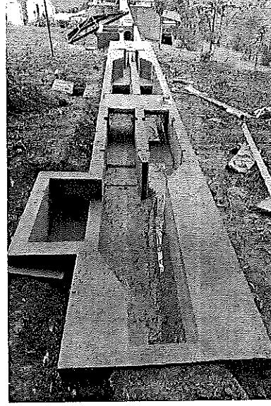
FOTOGRAFIA 11 Y 12: UNIDADES DE PRETRATAMIENTO RESANADAS Y PAÑETAS EN SU TOTALIDAD
