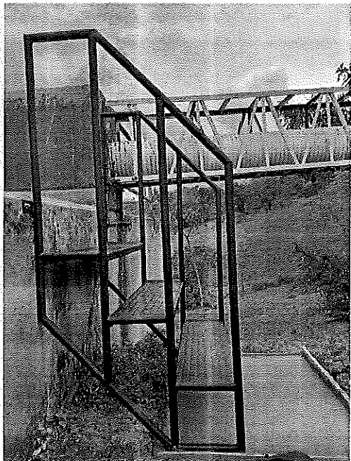
FOTOGRAFIA 7 Y 8: ESCALERA EN TUBERIA A.N. DIAMETRO 1" CALIBRE 16 LAMINA ALFAJOR DE 2.5 MILIMETROS.
