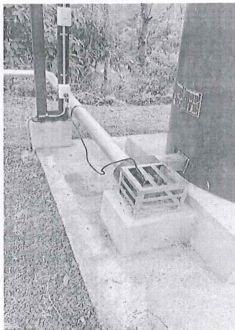
FOTOGRAFIA 15 Y 16: FILTRO PARA CONTROL DE OLORES. CON VENTILADOR CENTRIFUGO.
