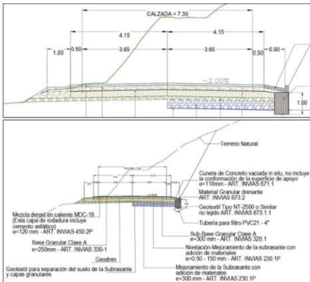
Ilustración 3 Sección típica en corte
