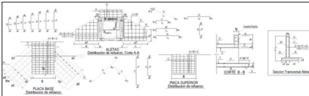
Ilustración 9 Box culvert de sección rectangular
