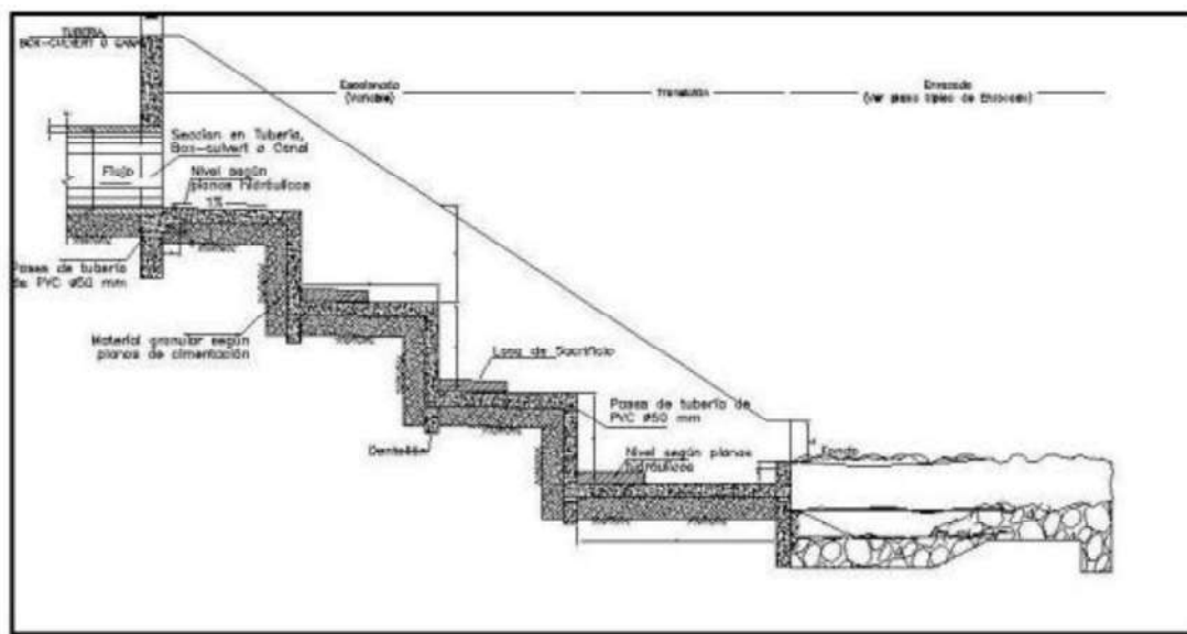
Ilustración 6 Estructura escalonada para la disipación de energía.
