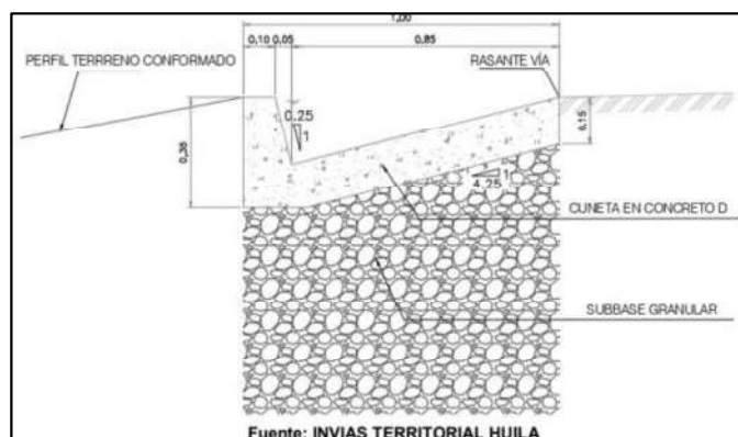
Ilustración 4 Detalle Transversal de la Cuneta.
