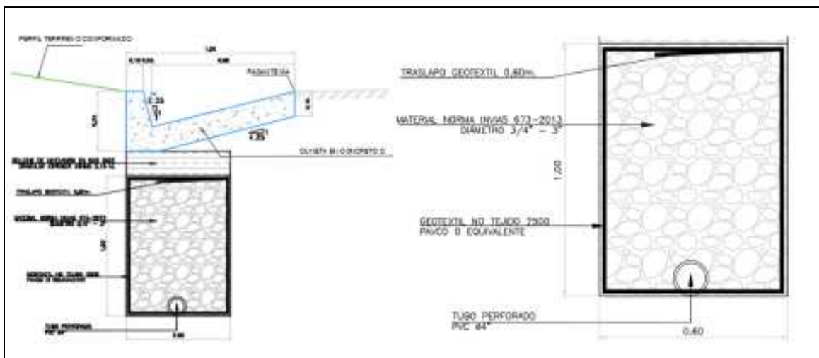
Ilustración 5 Sección Típica de Instalación del Filtro.
