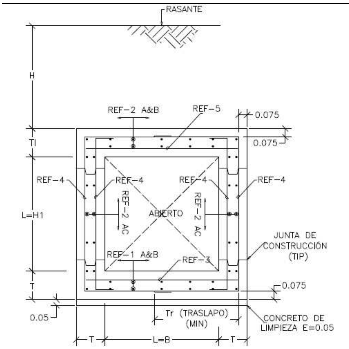
Ilustración 9 Box culvert de sección rectangular
