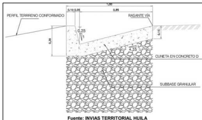
Ilustración 4 Detalle Transversal de la Cuneta.
