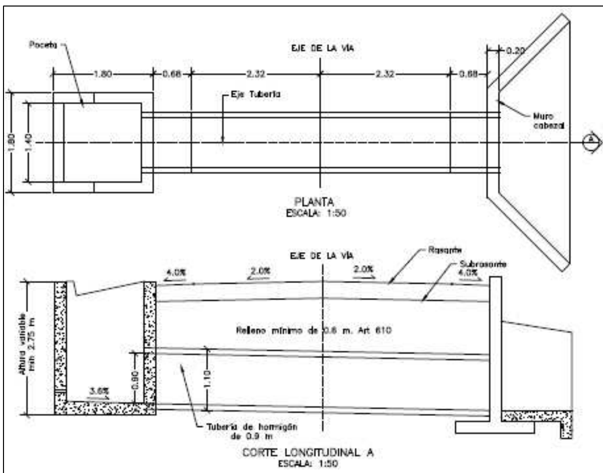
Ilustración 10 Esquema obras de drenaje transversales
