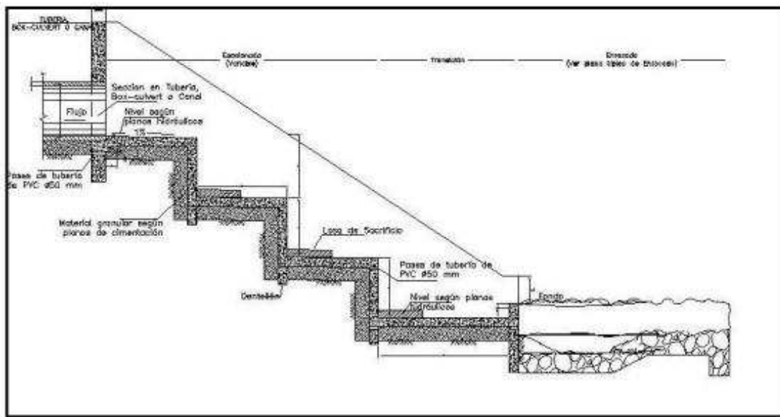
Ilustración 6 Estructura escalonada para la disipación de energía.
