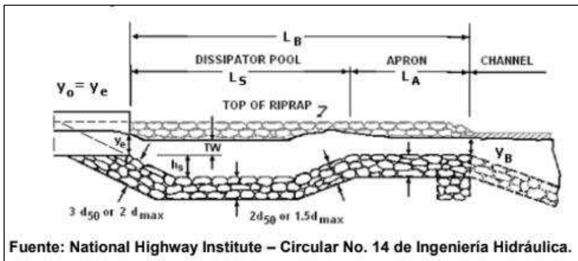
Ilustración 7 Perfil de Instalación de Enrocado de Protección.
