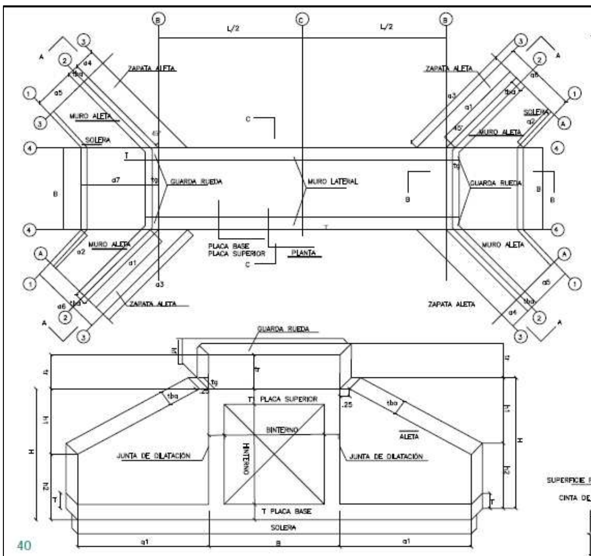
Ilustración 8 Box culvert de sección cuadrada
