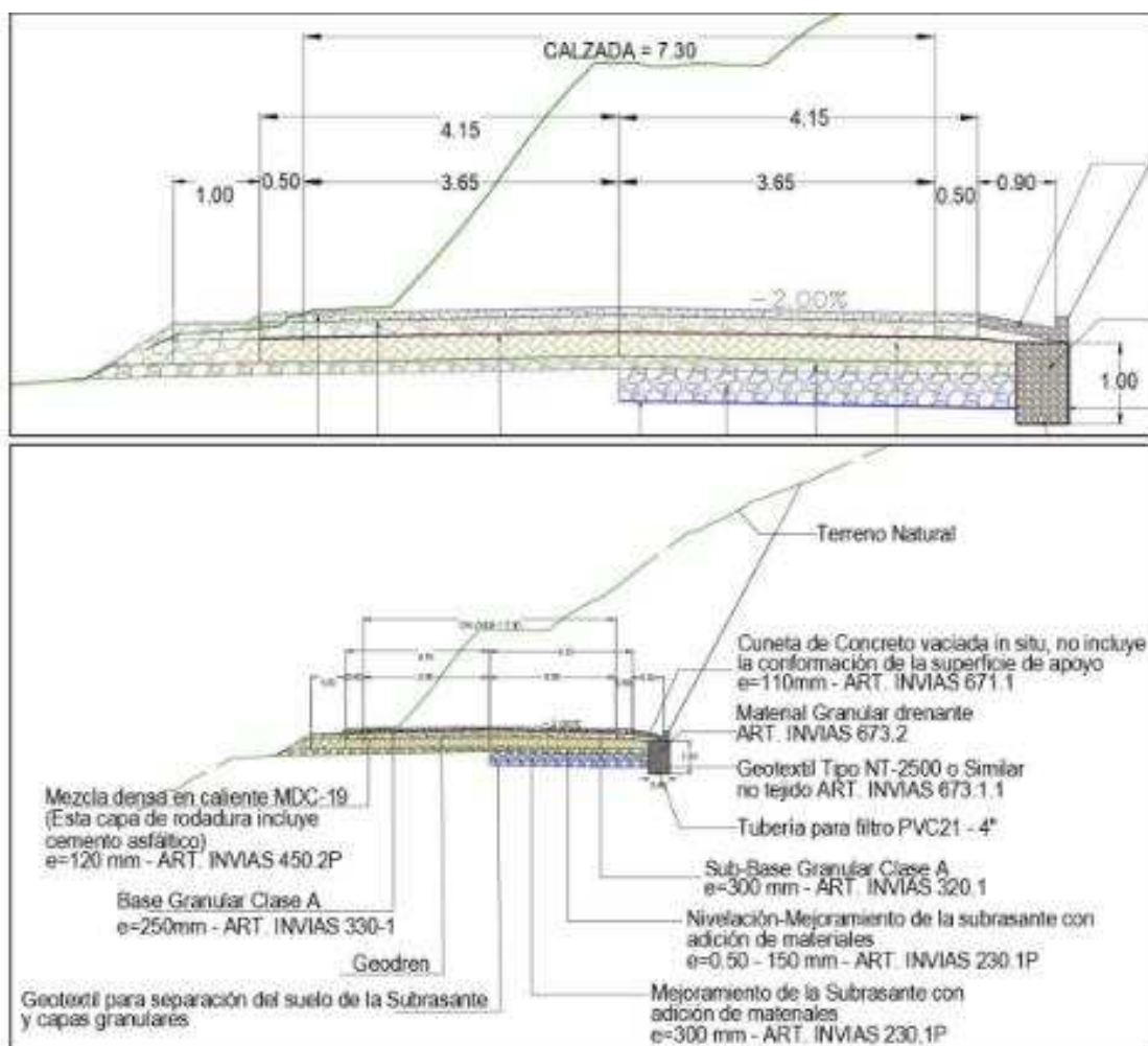
Ilustración 3 Sección típica en corte
