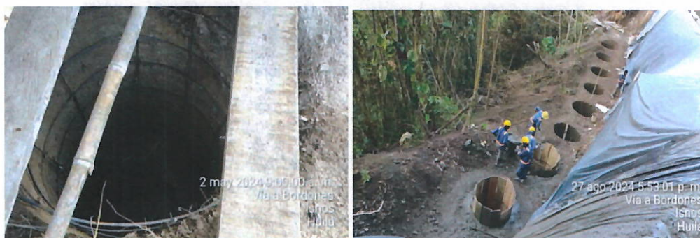
Ilustración 40 Camisa permanente en tramo 2
