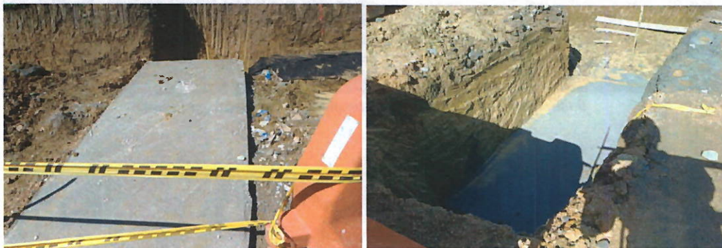
Ilustración 52 Conformación y renivelación en el zodme
