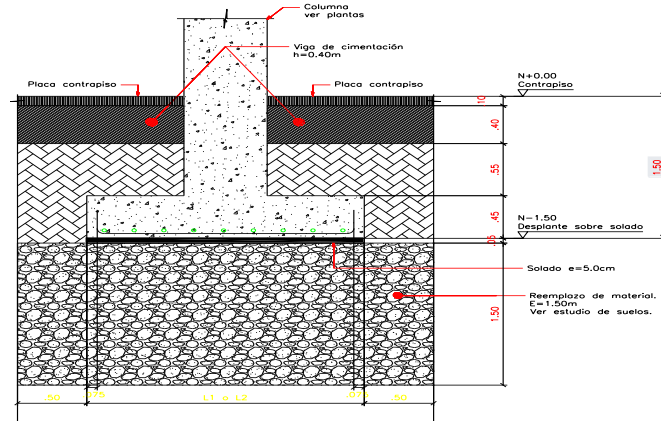
Detalle general de cimentación Acot. metros. Esc. 1:25
