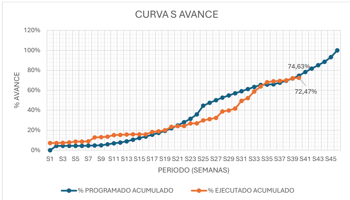
Gráfico 4 Curva S de avance físico
