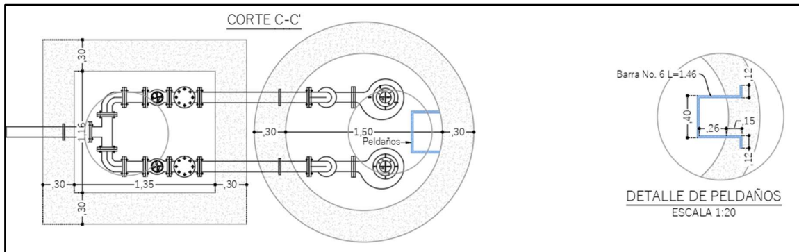
Ilustración 4 estación elevadora
