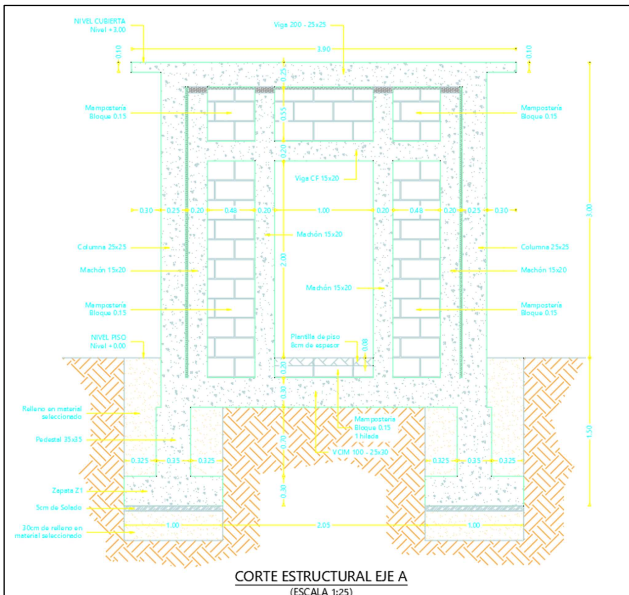
Ilustración 2 Estructura de caseta de bombeo
