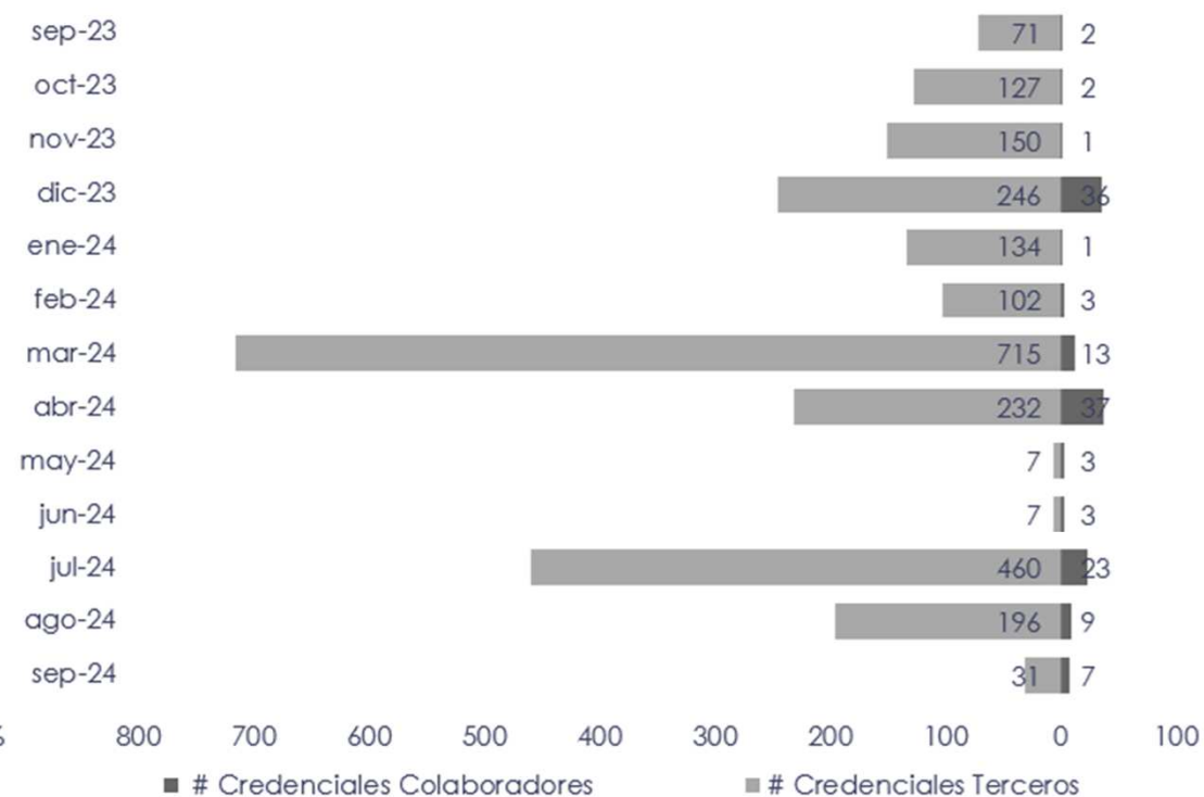
# de credenciales identificadas terceros VS colaboradores
