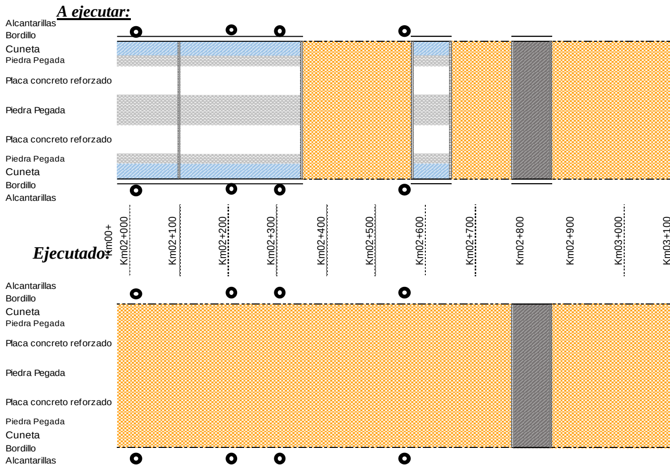
Figura 8. Avance de Obras Crucero - Palmas PR2+000 al PR3+100
