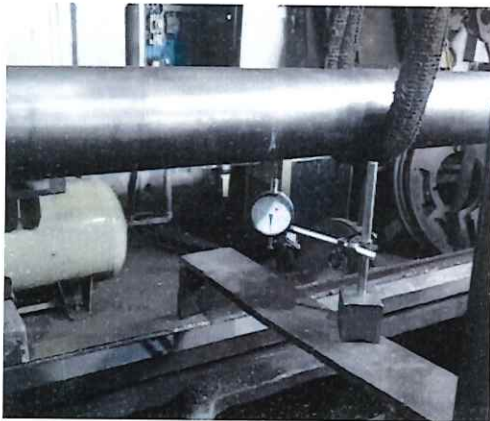
Imagen No. 21: Verificación del estado de las 12 secciones de las líneas de ejes de babor y estribor en torno.
