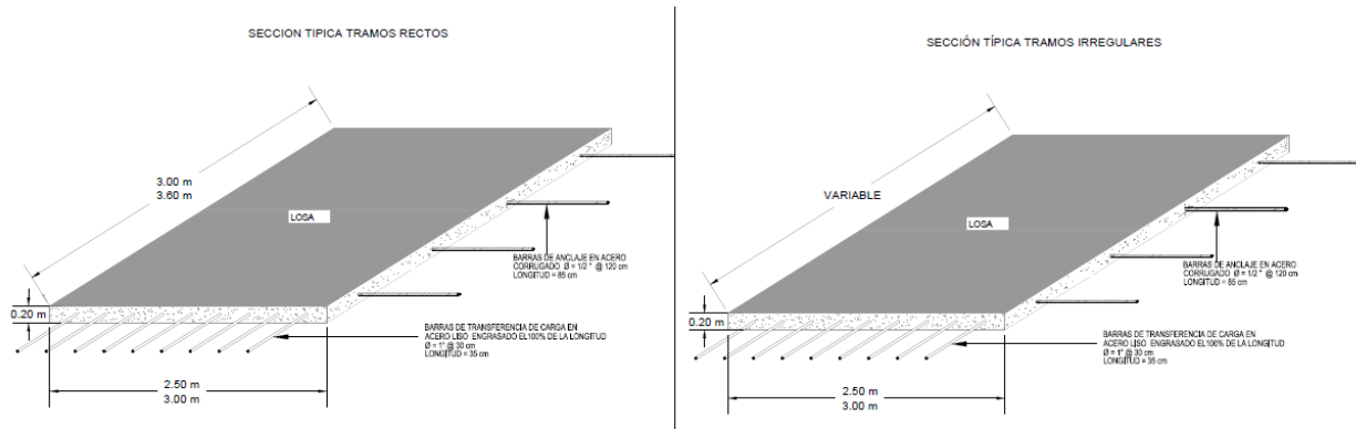
Figura 6. Sección típica
