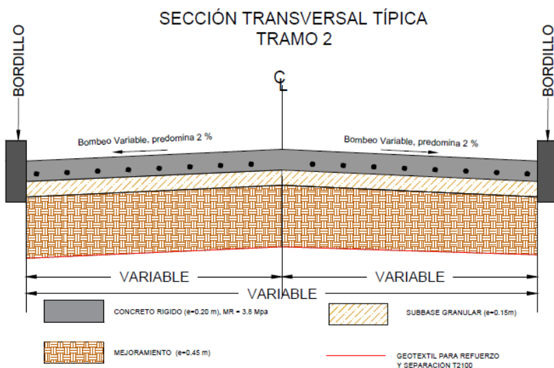
Figura 5. Tramo 2
