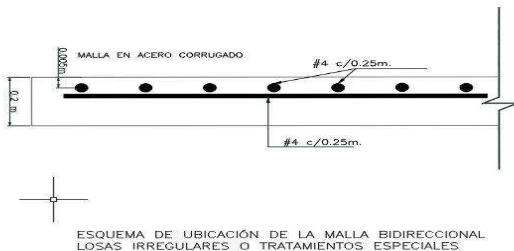
Figura 8. Detalle de Malla en Losas Irregulares
