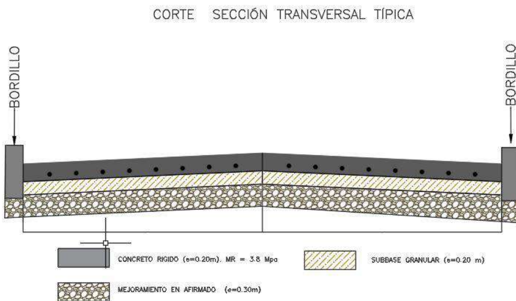
Figura 4. Sección Trasversal de la Vía Fuente:
