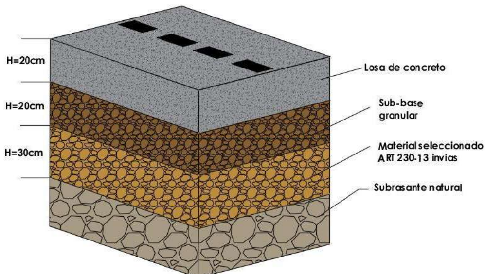
Figura 3. Espesores de capas Fuente: Diseños
