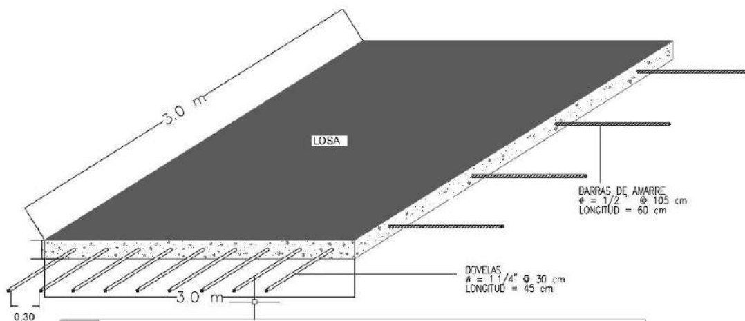
Figura 5. Sección Típica de Tramos Rectos Fuente:
