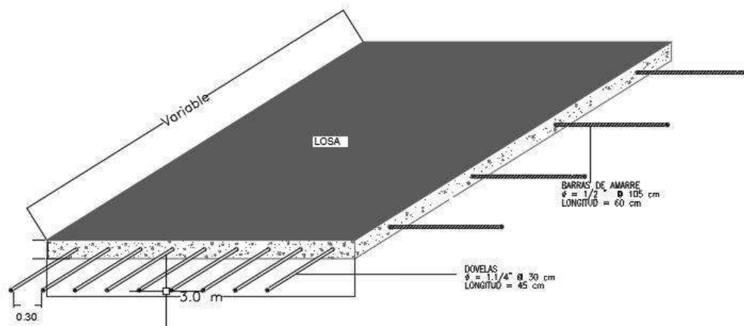
Figura 6. Sección Típica de Tramos Irregulares
