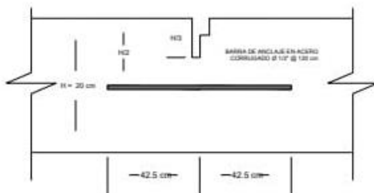
DETALLE CONSTRUCTIVO JUNTA LONGITUDINAL
