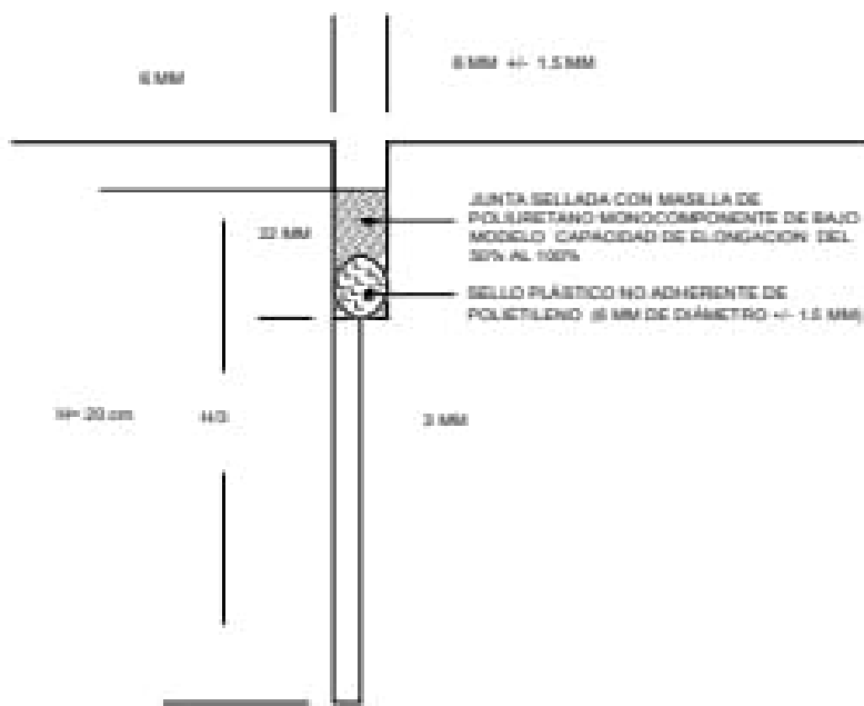
DETALLE CONSTRUCCION JUNTA LONGITUDINAL
