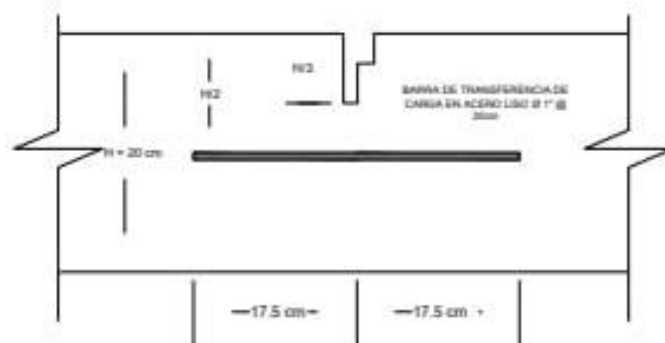
DETALLE CONSTRUCTIVO JUNTA TRANSVERSAL
