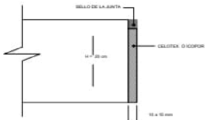
DETALLE CONSTRUCTIVO JUNTA DE EXPANSIÓN
