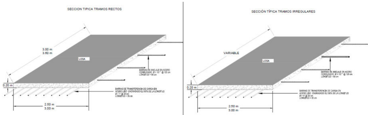
Figura 6. Sección típica
