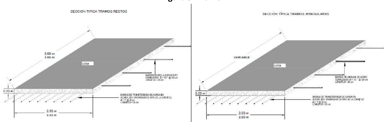
Figura 6. Sección típica
