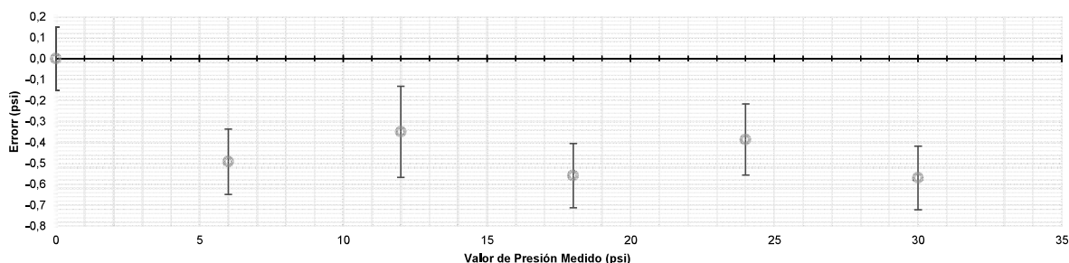
Figura 1. Gráfico de error de medición vs. valor de presión
