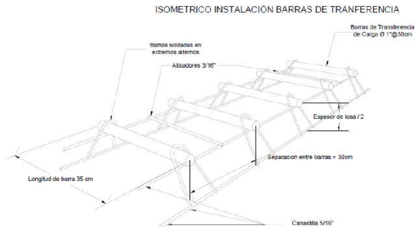
Figura 7. Canastillas de Instalación de barras de transferencia.
