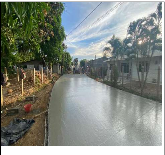
FOTO No. 56 Fundida de concreto en tramo T5 entre absc K0+190 a la K0+000
