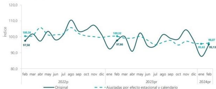
Gráfico 11. Índice de las actividades secundarias (base 2015) Serie original y serie ajustada por efecto estacional y calendario 2022 P - 2024 P (febrero)
