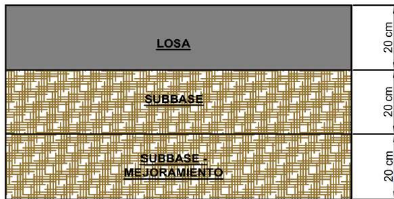
Imagen 7-2 Estructura de pavimento a construir tramo 2. Fuente, Autor
