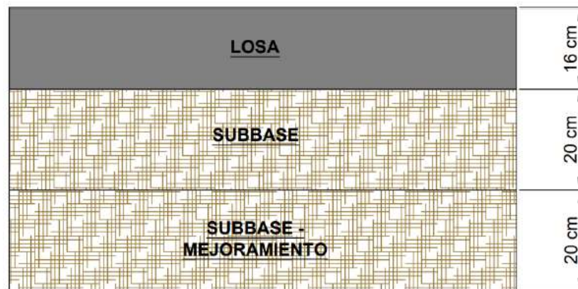
Imagen 7-1 Estructura de pavimento a construir tramo 1. Fuente, Autor
