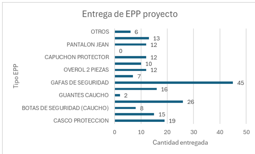
Grafica. Entrega de EPP en obra
