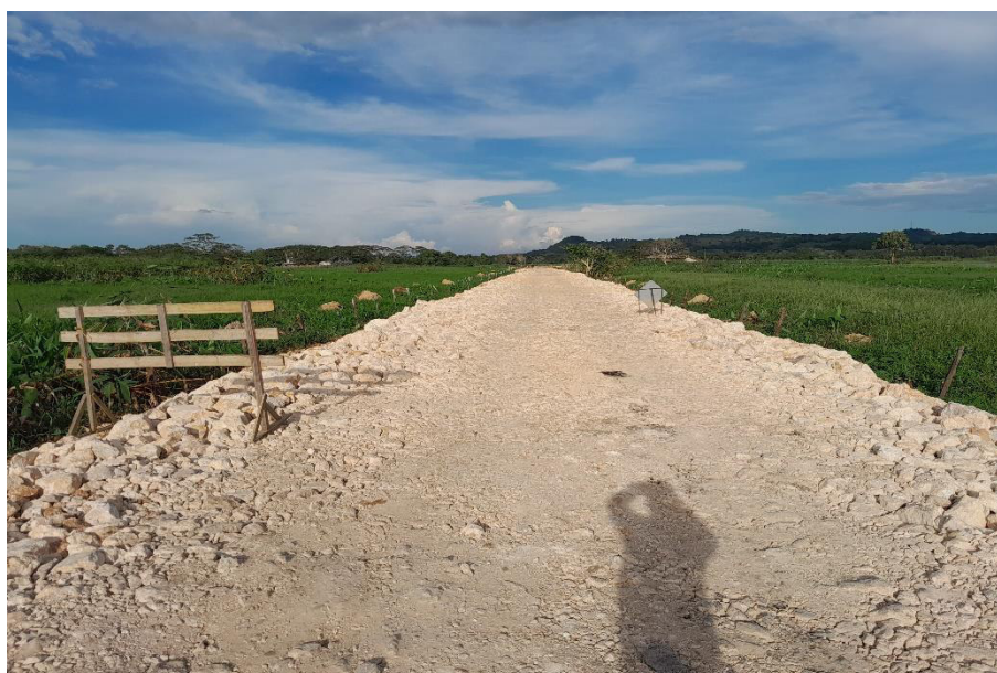
Fotografía N°10. Conformación de pedraplén en Km 4+600.
