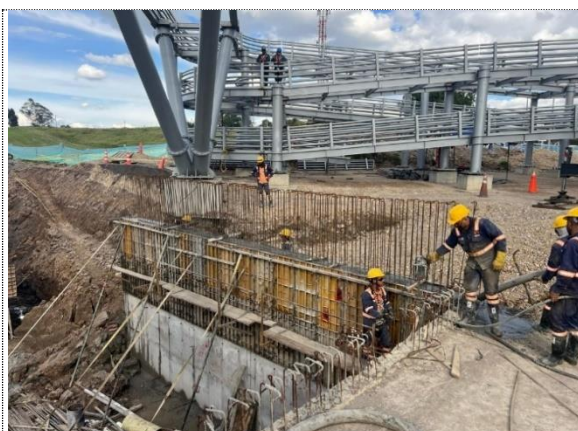
VARIANTE ZIPAQUIRÁ, OBRA No 19, FUNDIDA DE 4ta SECCIÓN DE VÁSTAGO DE MURO DE CONTENCIÓN
