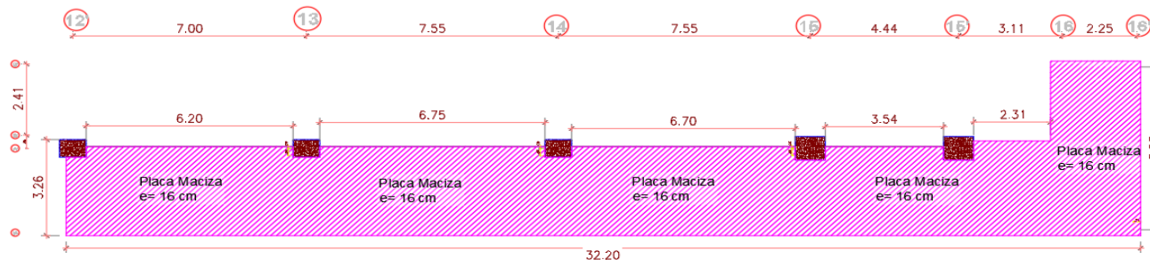
PLANTA PRIMER TRAMO RAMPA
