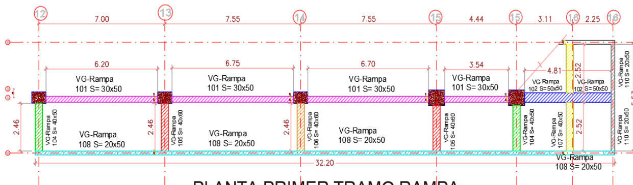
PLANTA PRIMER TRAMO RAMPA
