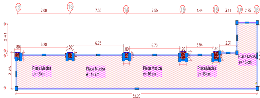
PLANTA PRIMER TRAMO RAMPA
