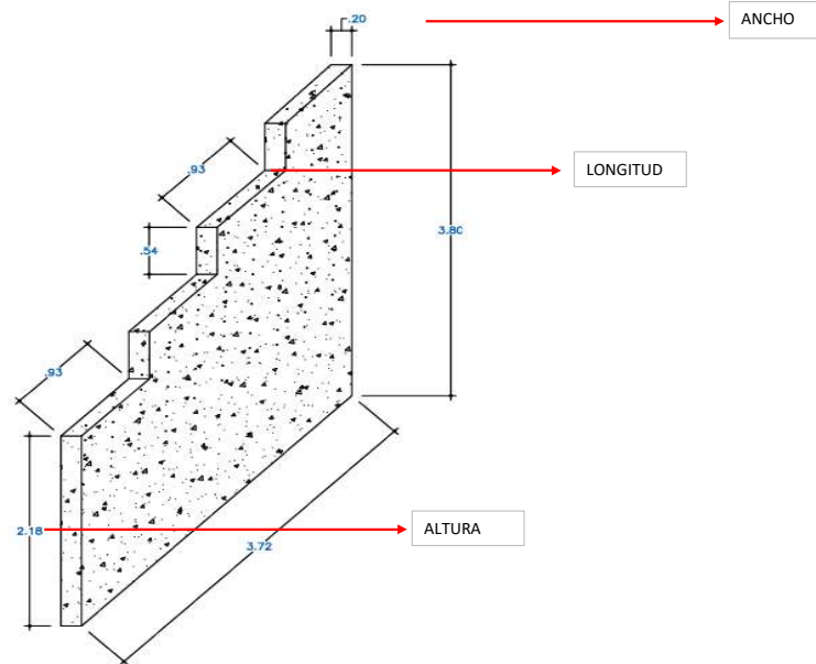
Muro cortina para base de graderías del edificio A entre ejes 3 y 4, entre las alturas 8.02 metros y 12.42 metros ESCALA 1:25
