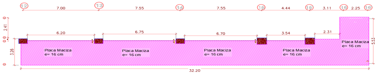
PLANTA PRIMER TRAMO RAMPA
