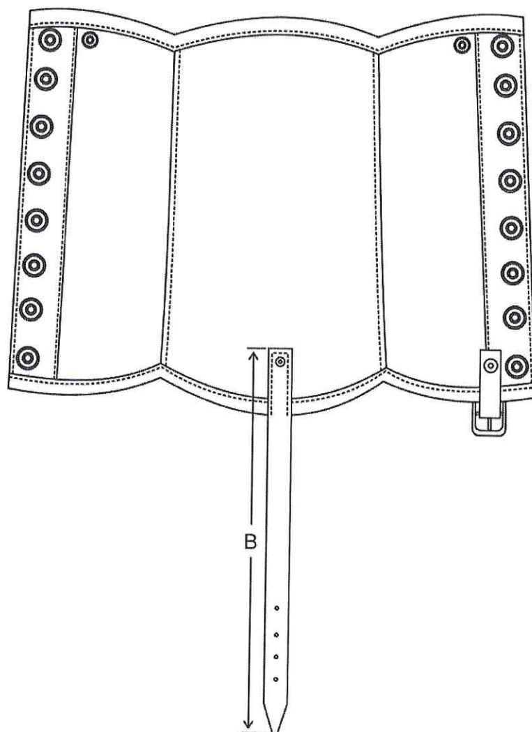
Figura 2. Vista posterior de la polaina
