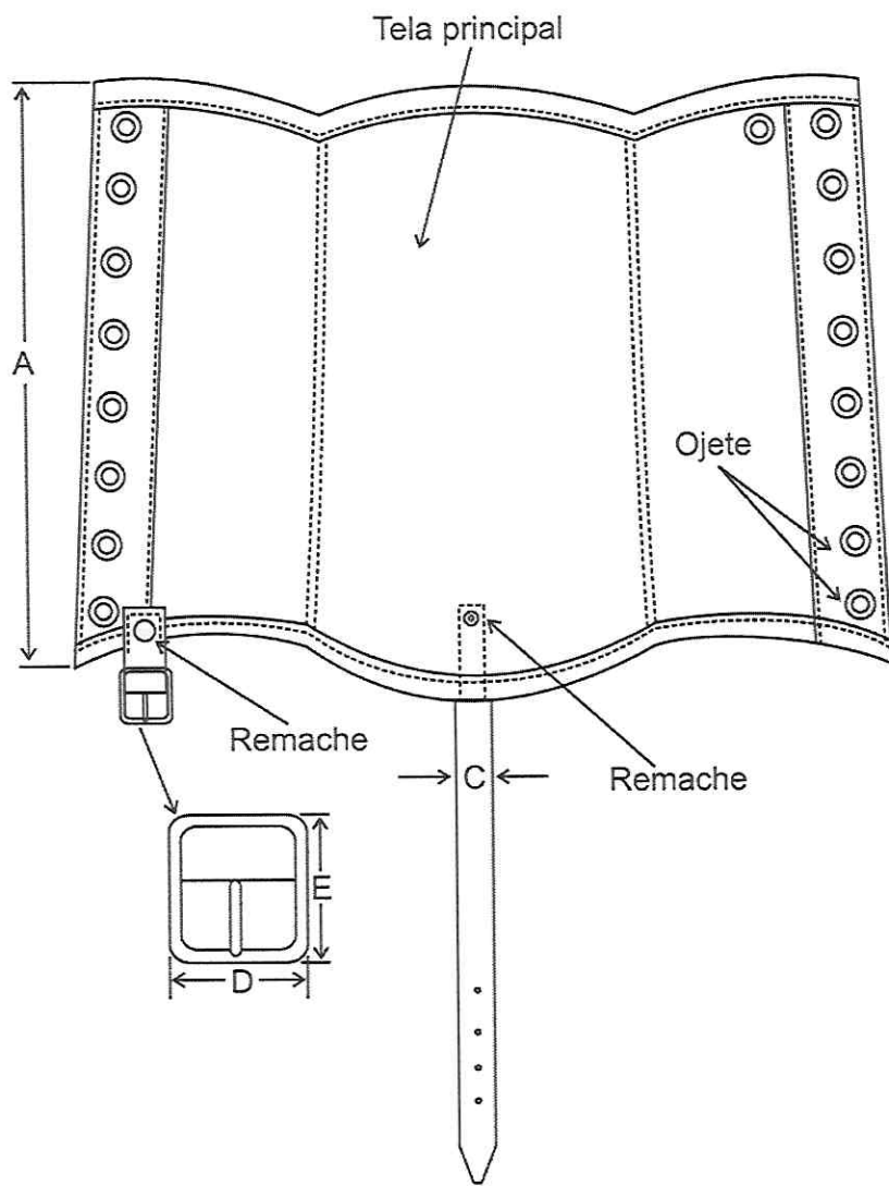
Figura 1. Vista anterior de la polaina
