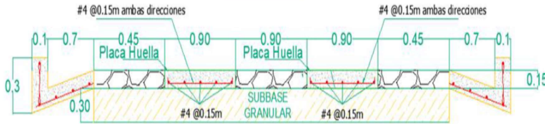
Imagen 6. Vol. I Estudio y diseño estructura de placa huella
