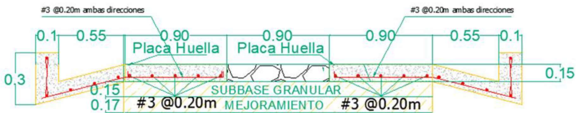
Imagen 9. Tomado del Diseño de Estructura de Placa Huella de OR Construcciones e Ingeniería SAS
