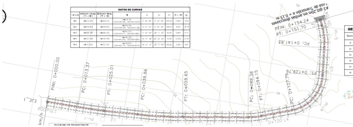
Imagen 20 Tomado Diseño Geométrico V1 OR Construcciones e Ingeniería SAS
