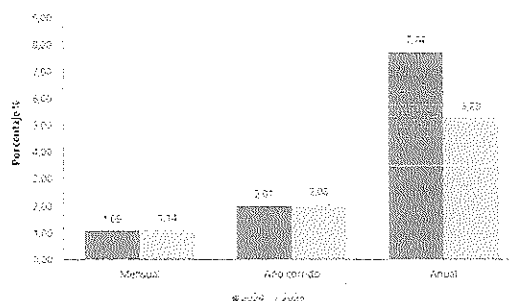
Gráfico 1. IPC Variaciones Total Nacional Febrero 2024 - 2025
