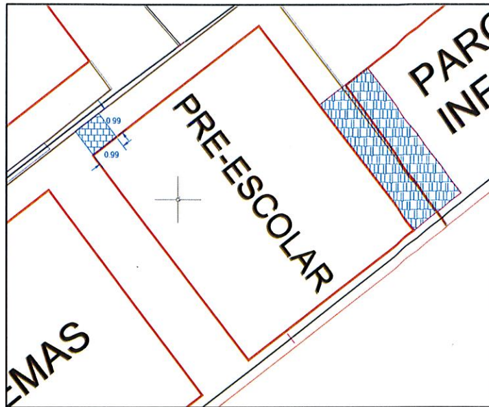
Figura 9. Zona de demolición de piso para instalación de bajante a cárcamo
