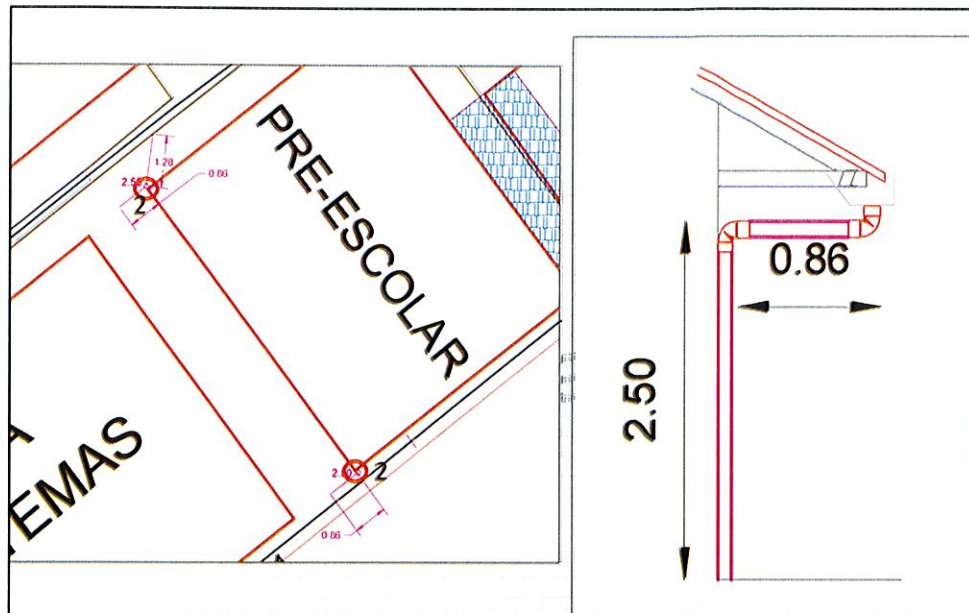
Figura 8. Ubicación de bajantes y geometría de las mismas para descarga en cárcamos a ejecutarse
