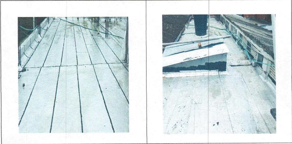
IMPERMEABILIZACIÓN DE PLACA DE CUBIERTA, CON IMPERMEABILIZANTE DE ALTA RESISTENCIA (EMULSION Y MANTO ASFALTICO EN CALIENTE) QUE EVITA TOTALMENTE LA PENETRACIÓN DE HUMEDAD Y ABSORBE LOS MOVIMIENTOS ESTRUCTURALES.
