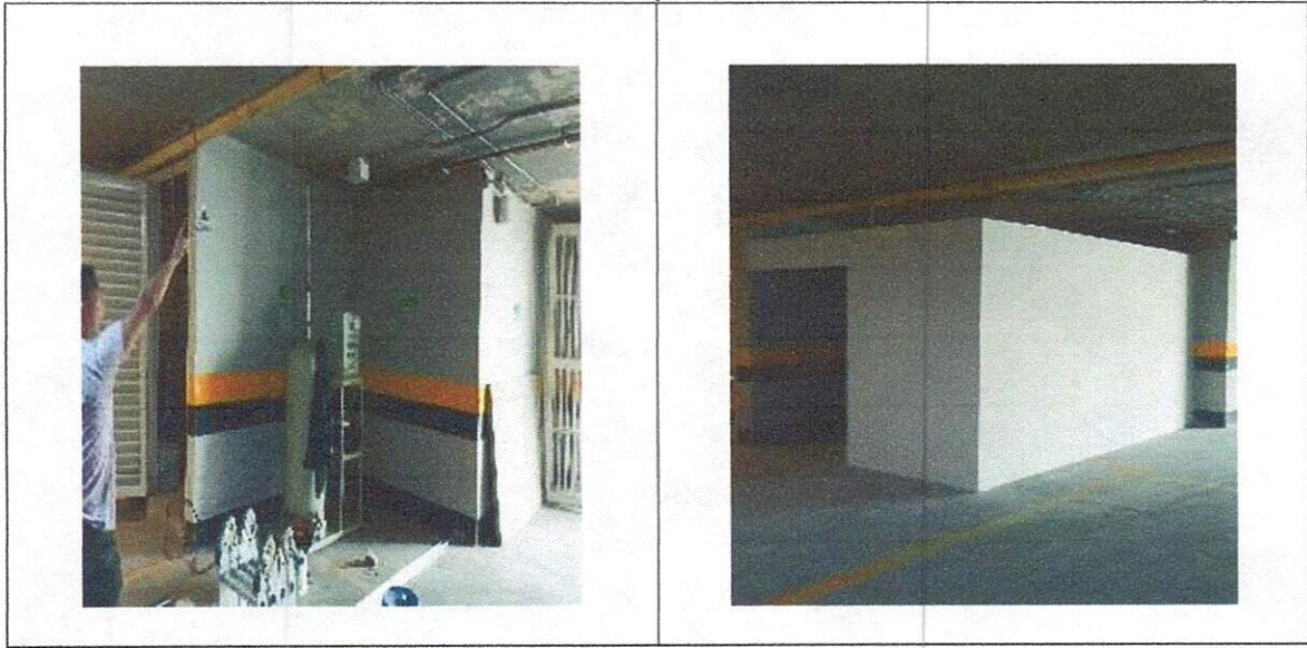
MURO DRYWALL DOBLE CARA 0.12 M (INCLUYE VINILO TIPO 1 A DOS CAPAS)
