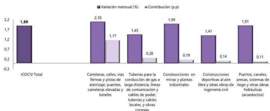
Variación mensual y contribución del ICOCIV según tipos de construcción Total nacional Fuente: DANE, ICOCIV - DANE - Índice de Costos de la Construcción de Obras Civiles (ICOCIV)
