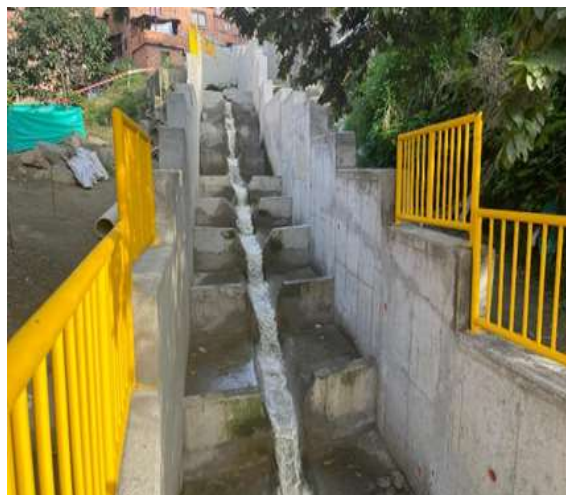
Foto 4 VISTA DEL CANAL ABIERTO REFORZADO AGUAS ARRIBA
