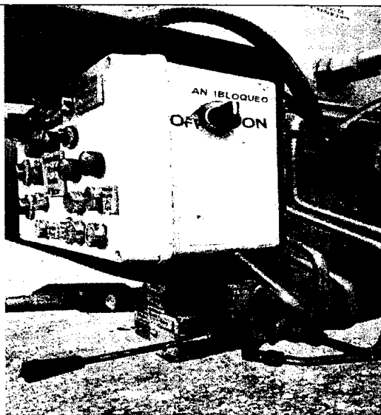
Figura No.8 REVISIÓN TABLERO DE MANDOS
