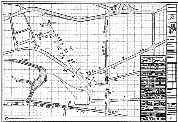
Imagen Plano diseño proyectado ordenamiento vial san Antonio.
