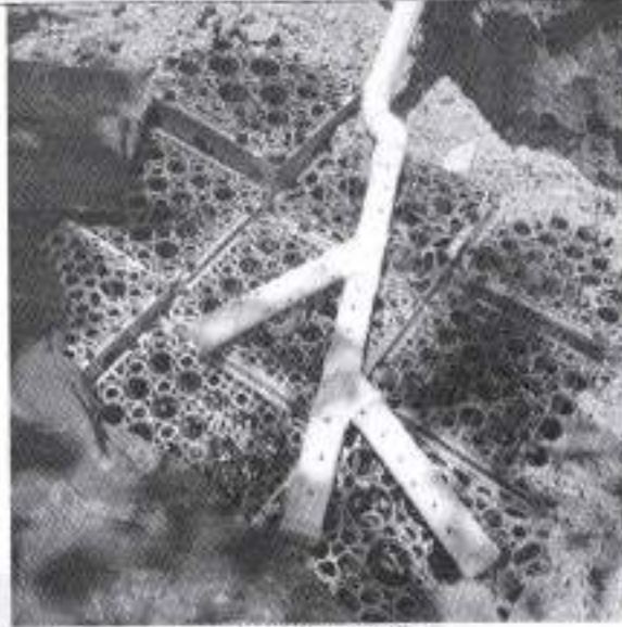
Imagen 9. Detalle de la tubería de PVC.
