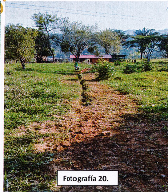
Fotografía 17-20. Relleno en material seleccionado de la excavación compactado para línea de gas.
