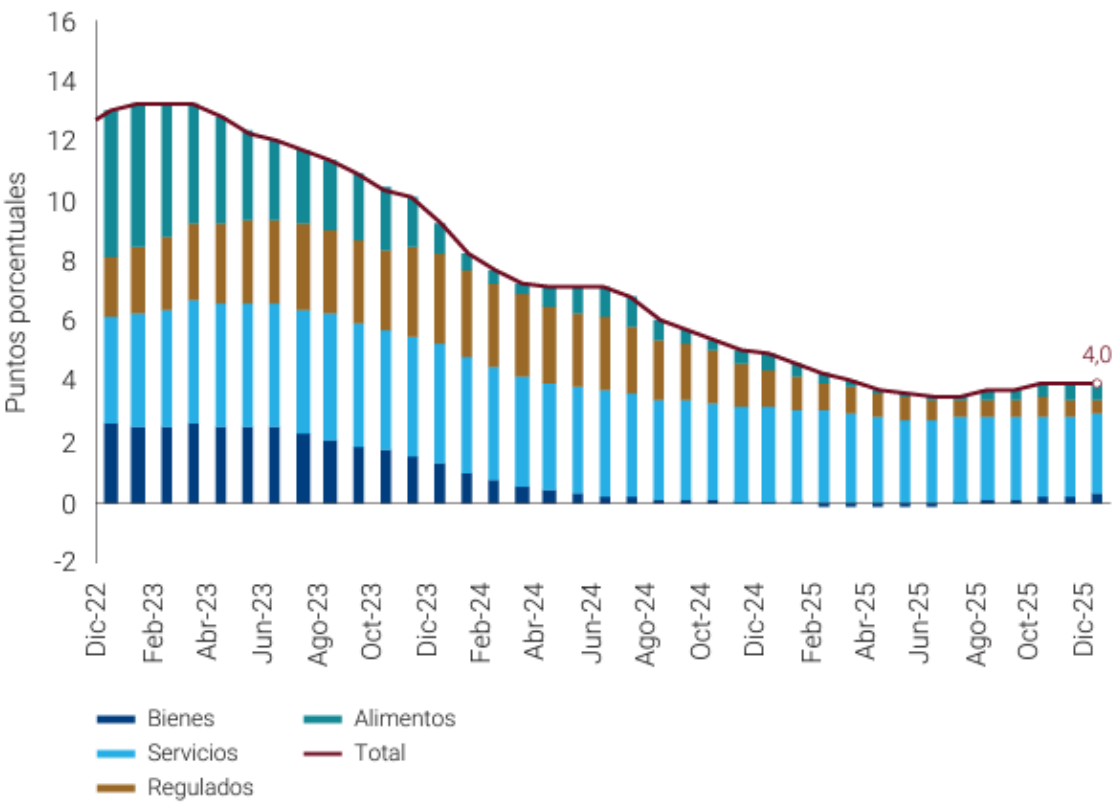
Gráfico 10 APORTES A LA INFLACIÓN ANUAL
