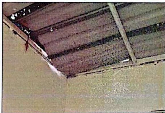
Correas metálicas soporte de Cubierta
