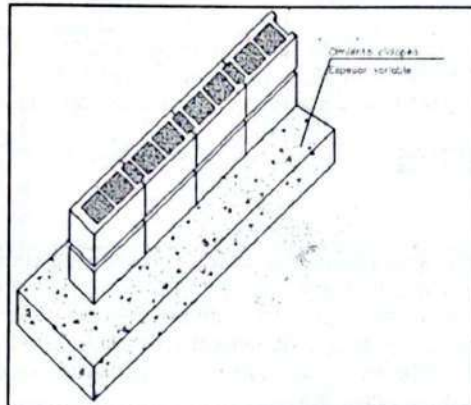
Cimientos típicos para muros medianeros
