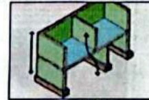
Figura 6.30: Vulnerabilidad media: irregularidad en altura.
