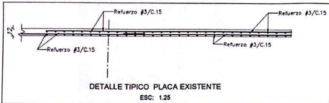
Armadura que se presume tiene la paca
