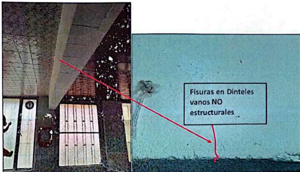
Muros perimetrales Primer piso
