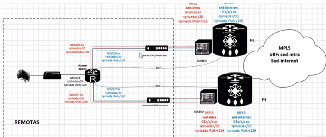
Ilustración 7 Diseño core Claro
