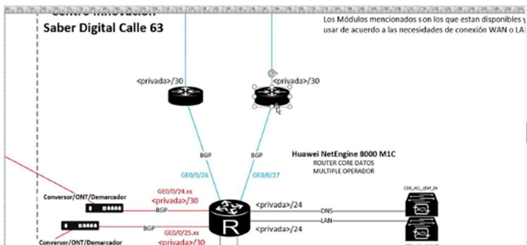
Ilustración 4 Diseño general conexión Core Claro
