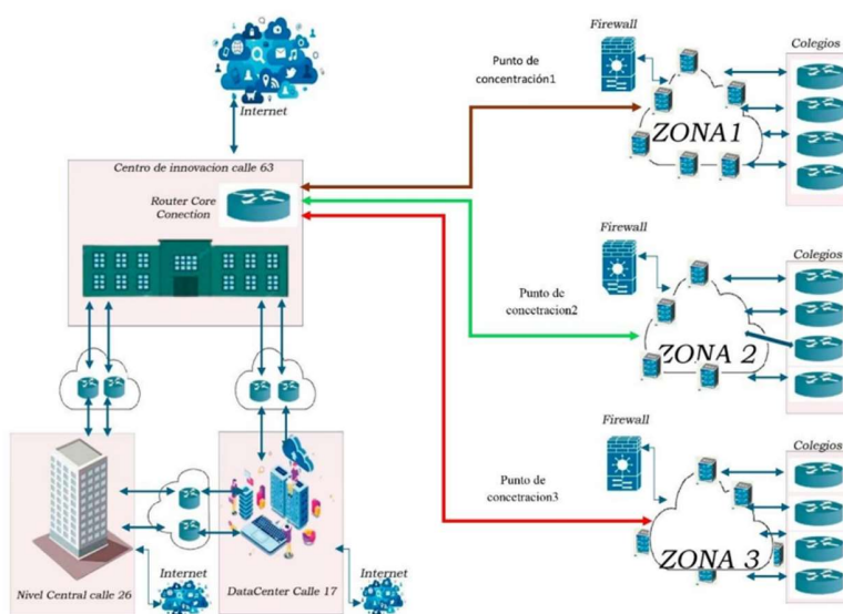
Ilustración 1 Diseño aprovisionamiento sedes
