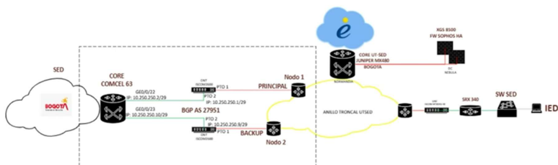
Ilustración 5 Interconexión router claro
