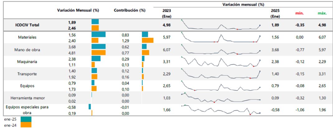
Gráfico 15. Variación mensual y contribución del ICOCIV, por grupos de costos
