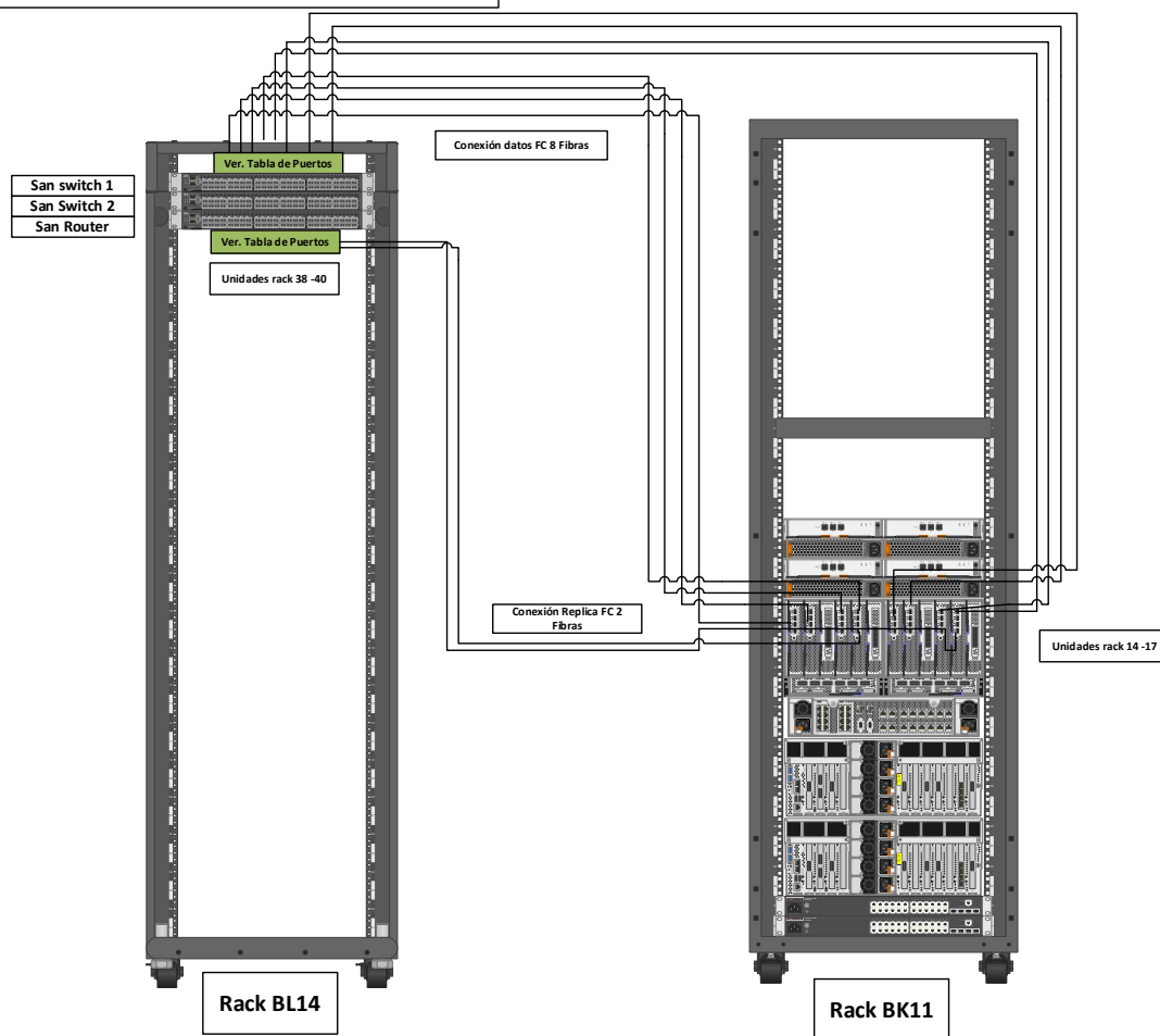
Diagrama de Conexión FC DS9850 – SAN SWITCH
