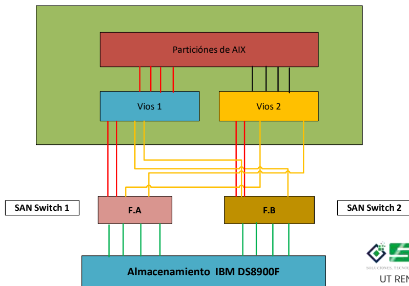
Diagrama de Conexión de IBM Power10 a SAN Switch Dual Vioserver
