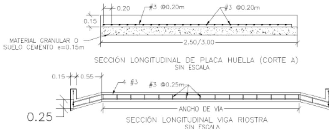
Figura 3 Esquema placa huella de longitud losa y acero transversal
