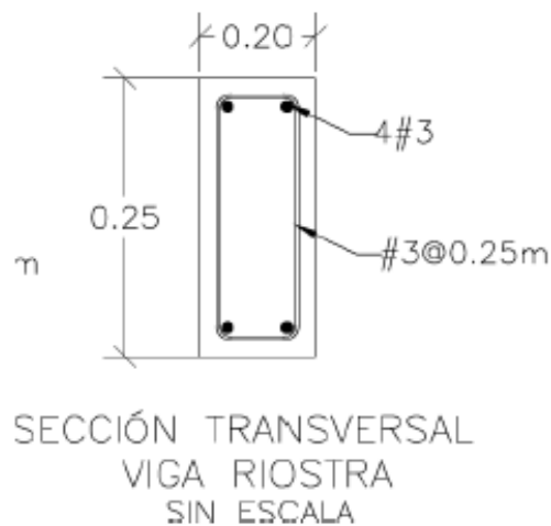
Figura 4 Esquema Sección viga riostra
