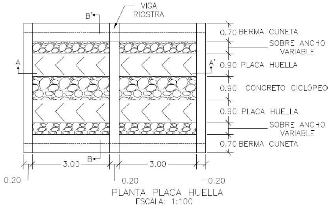
Figura 2 Esquema Vista en planta
