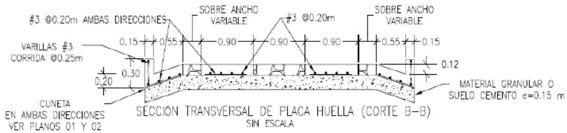
Figura 1 Esquema placa huella sección transversal cuneta
