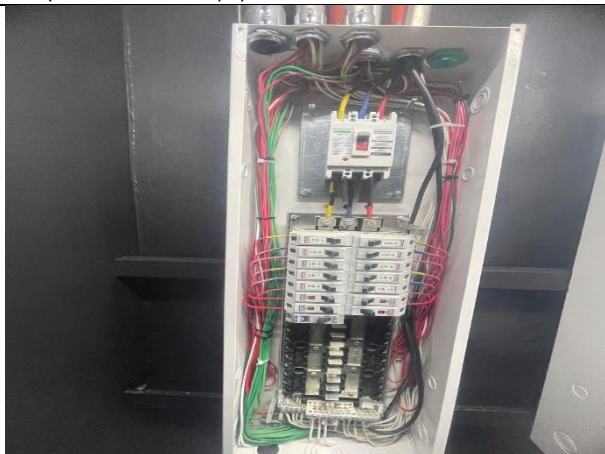
8. instalación acometida eléctrica para pantalla 163 (8)
