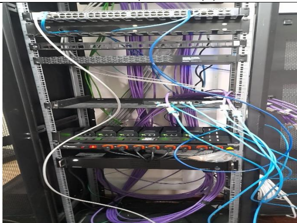
28. Instalación equipos en rack (2)
