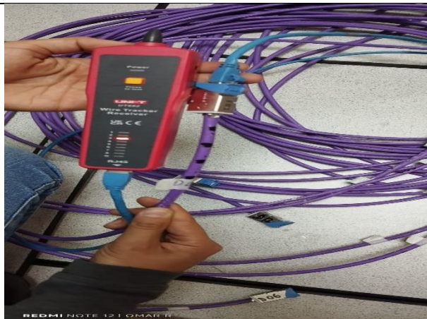
27. verificación puntos de red CS1
