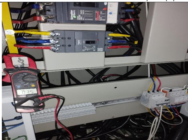
6. Conexión a tablero eléctrico 4 piso (6)
