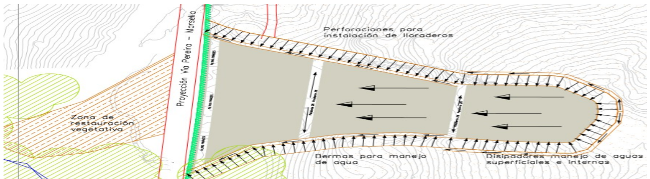
Ilustración 2. Modelación Cárcava Deslizamiento Muro Tablestacado.
