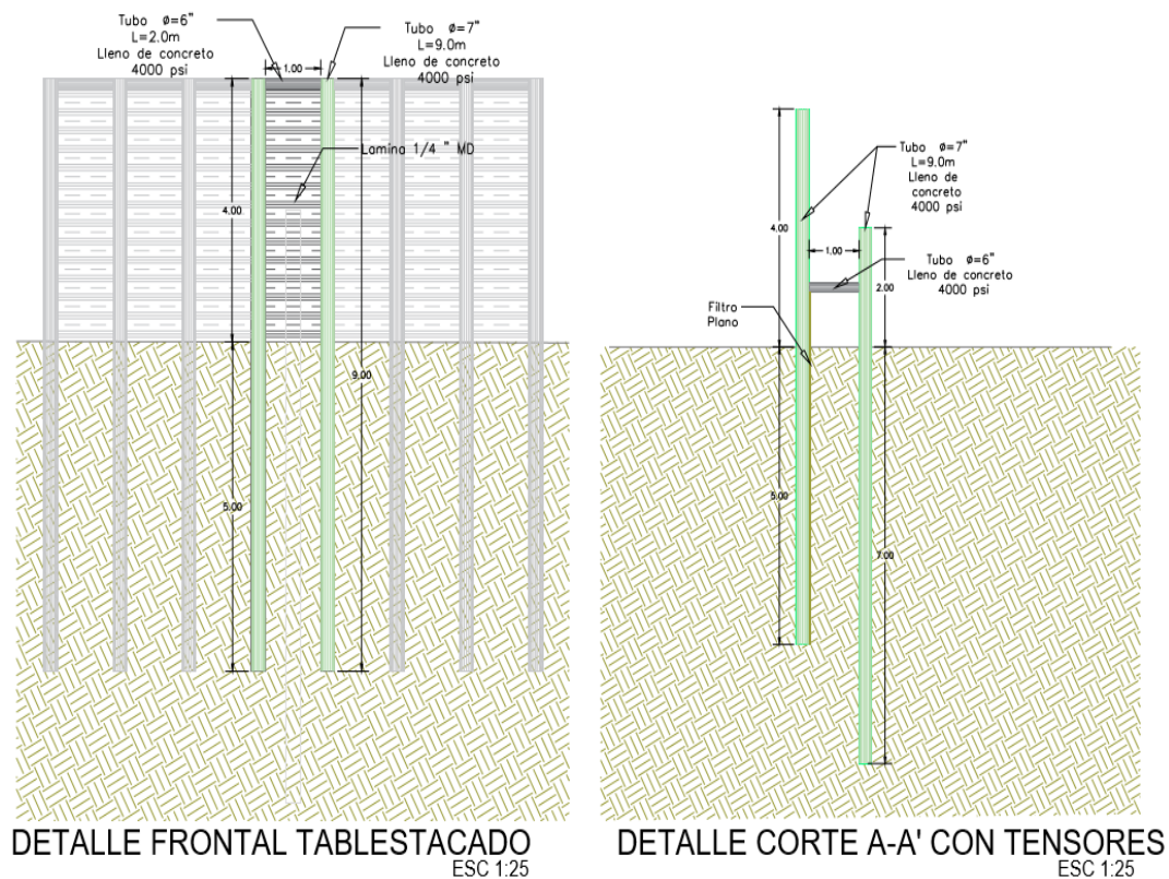
Ilustración 3. Detalles de Muro Tablestaca Marsella Vereda Oriental K-19.
