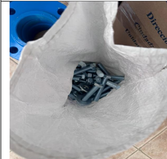
TORNILLO, TUERCA Y ARANDELA 5/8" POR 3.1/2
