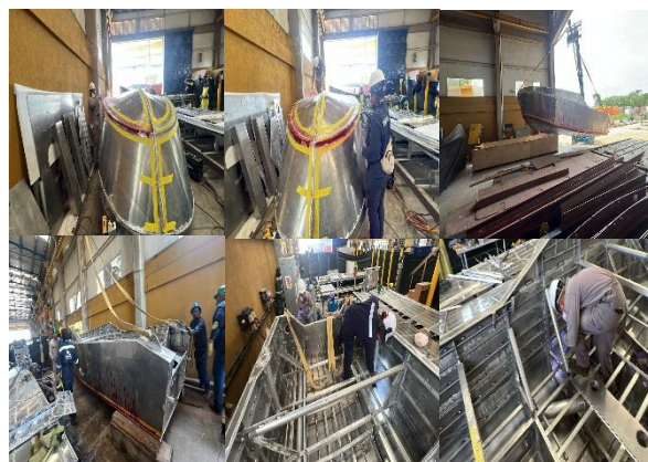
Foto No. 79 a 84 – bote 2 ensayos no destructivos y volteo
