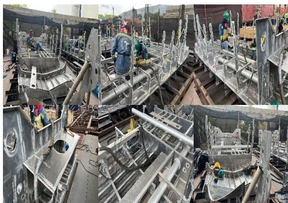
Foto No. 47 a 52 – bote 4 refuerzos, cuadernas vagras tuberías
