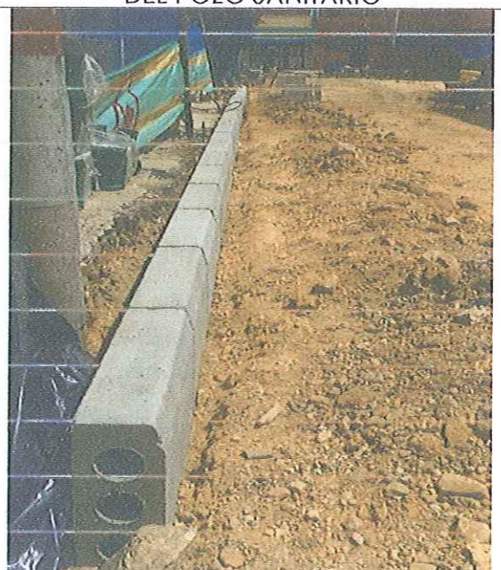
INSTALACIÓN DEL SARDINEL PREFABRICADO A-10
