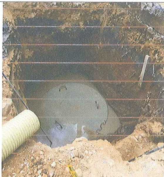
INSTALACIÓN DE LA PLACA DE FONDO DEL POZO SANITARIO
