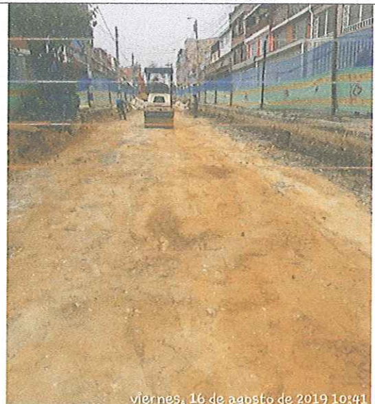
INSTALACIÓN Y COMPACTACIÓN DE LA SUBBASE GRANULAR
