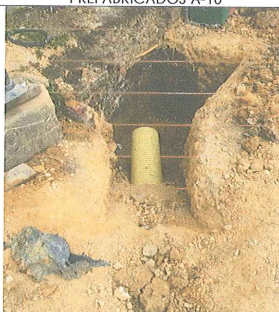
INSTALACIÓN DE TUBERIA NOVAFORT DE 10" PARA SUMIDEROS
