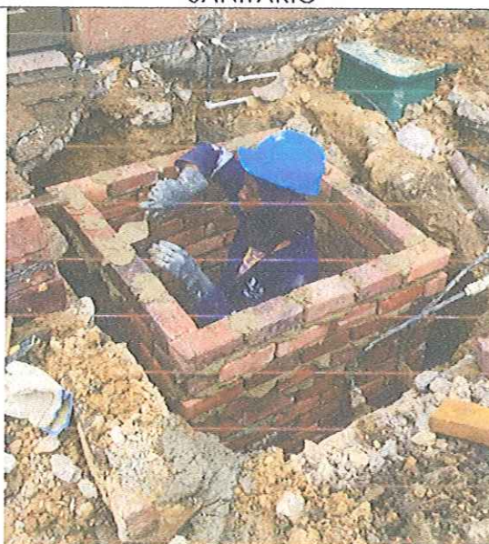
CONSTRUCCIÓN DE CAJAS DE INSPECCIÓN
