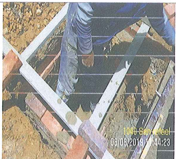
CONSTRUCCIÓN CAJAS DE INSPECCIÓN DEL JARDIN
