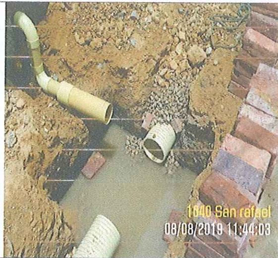
INSTALACIÓN DE TUBERÍA EN NOVAFORT PVC DESAGUE DEL JARDIN
