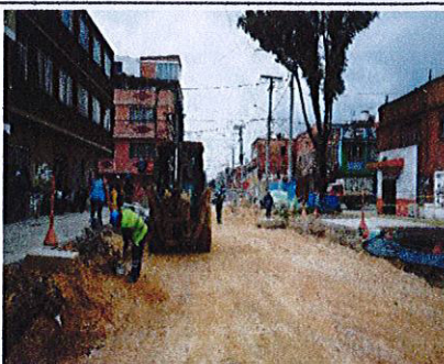
FOTOS Nos 4 y 5 CIV 160028646 Suministro e instalación material para segunda capa de subbase
