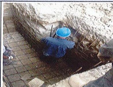
Foto 3. Armado de refuerzo sumideros combinados CIV 16001256
