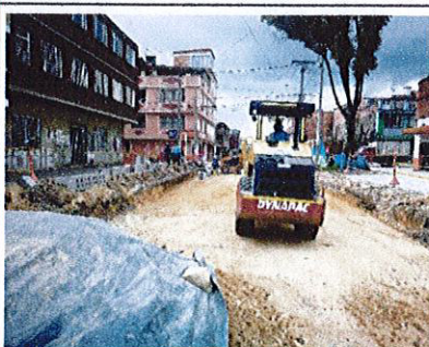
Foto 9. Compactación capa de renivelación en subbase. CIV 16002846
