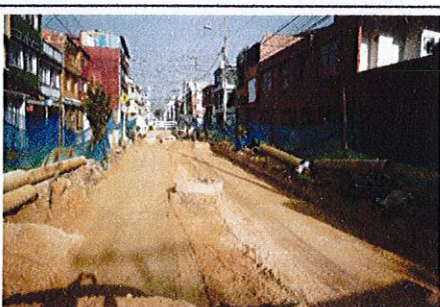
FOTO No. 9 CIV 16002769 Conformación primera capa de subbase.
