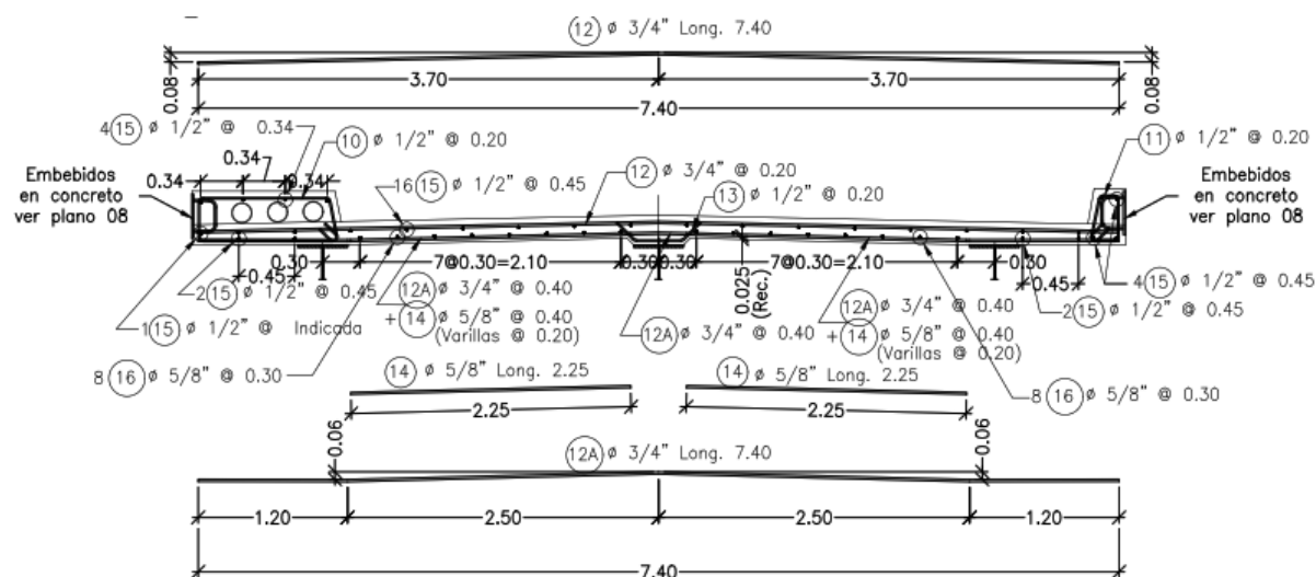
REFUERZO TRANSVERSAL TÍPICO LOSA (LOS)
