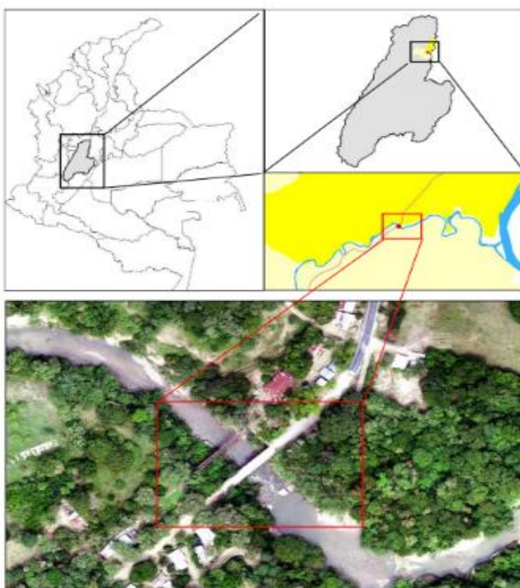
Figura No. 2. Localización Puente sobre el Río Venadillo en el corredor vial Palobayo – Ambalema Fuente: Estudios y diseños para la construcción del puente vehicular sobre el río Venadillo ubicado en el corredor vial Palobayo - Ambalema en el departamento del Tolima
