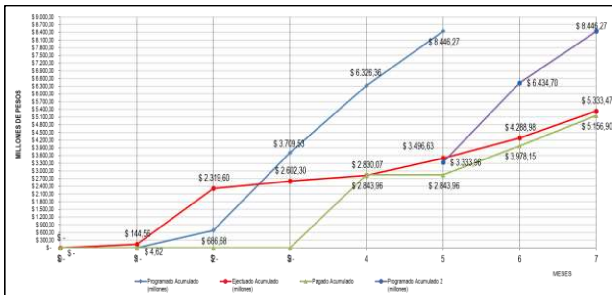
Imagen 6. Curva "S" del proyecto mes a mes.
