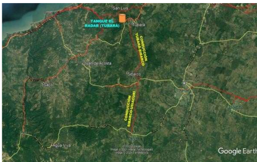
Imagen 3. Sistema de abastecimiento al municipio de Usiacurí. Fuente: Elaboración Propia con imágenes de Google Earth
