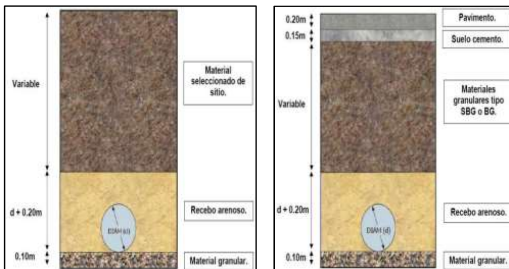
Imagen 7. Sección Típica instalación en Zona verde y Sección Típica Vías.
