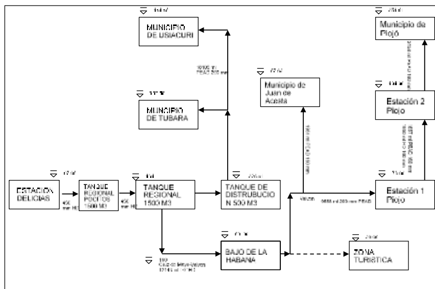
Figura 2. Esquema de componentes del Acueducto Regional Costero. Fuente: Anexo Técnico Contrato de Obra
