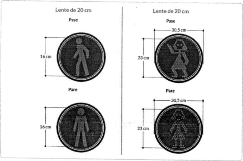
Figura 4-24. Simbología empleada en semáforos peatonales
