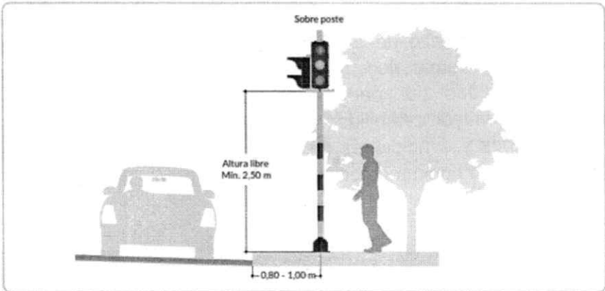
Figura 4-12. Semáforo soportado en poste pedestal
