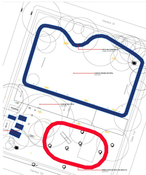
Grafica 1: Planta General de implantación escenario deportivo Santa Anita.
